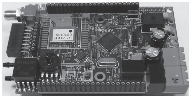
3. ábra. Az AERObot 5.0 alaplapp
